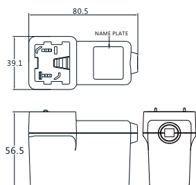
AC Plug-US
