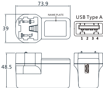
AC Plug-US
